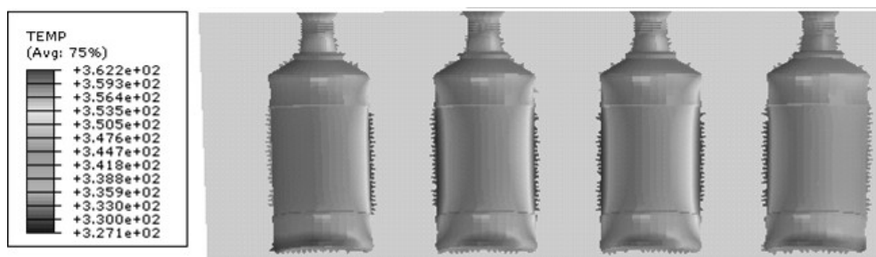
Rys. 3: Rozkład temperatury w gniazdach formy modelu nr 1 w 10 sekundzie symulacji (opracowanie własne)
