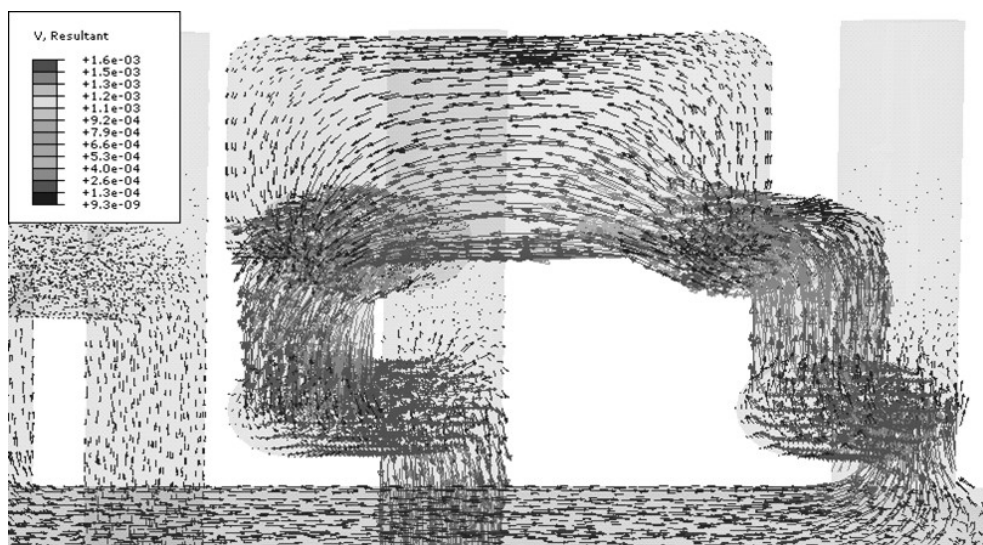
Rys. 2: Przepływ płynu w kanałach chłodzących w sekcji szyjki w trzeciej sekundzie symulacji modelu nr 1 formy obecnie produkowanej w Przedsiębiorstwie (opracowanie własne).
