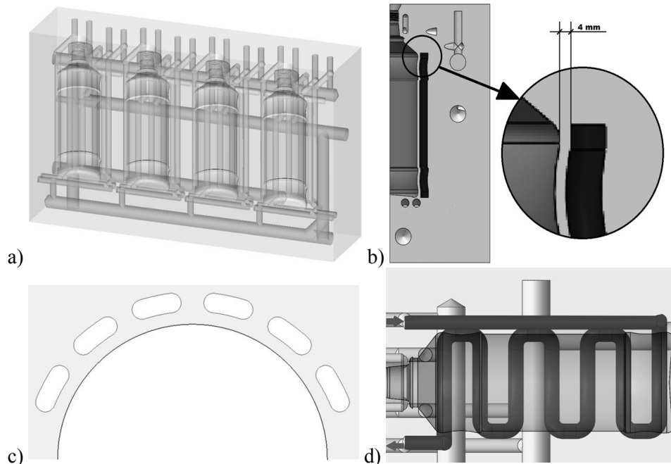
Rys. 1. Modele konstrukcji formy wykorzystane w badaniu (opracowanie własne) a) model 1 – uproszczona konstrukcja formy produkowanej przez Przedsiębiorstwo, b) model 2 –zbliżenie przebiegu kanału chłodzącego do profilu gniazda formującego butelki, c) model 3 – zmiana przekroju poprzecznego kanałów układu chłodzenia, d) model 4 – zmiana długości kanałów oraz kierunku przepływu chłodziwa.
